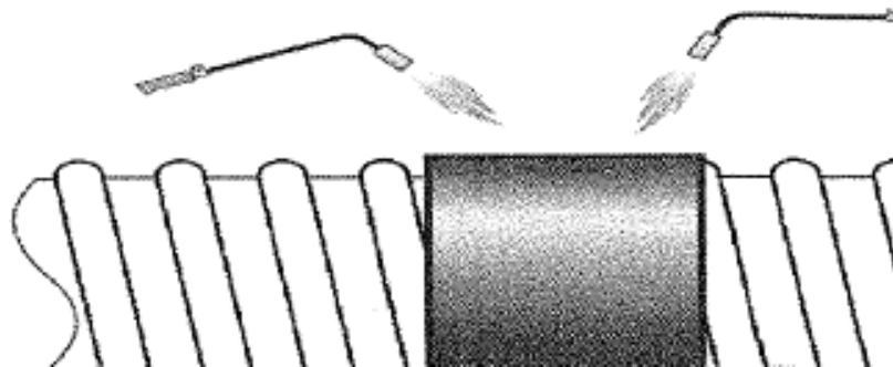
Рисунок 6.3 - Усадка муфты с помощью двух горелок
