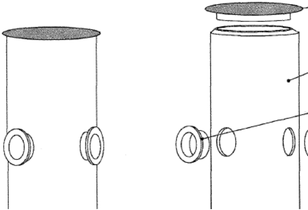
1 - полимерный люк; 2 - резиновая уплотнительная муфта; 3 - база-шахта; 4 - полимерный люк Рисунок 5.8 - Элементы модульного дренажного колодца
