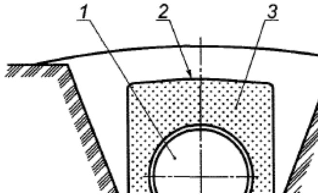
1 - трубопровод; 2 - полимерный контейнер; 3 - грунт засыпки
