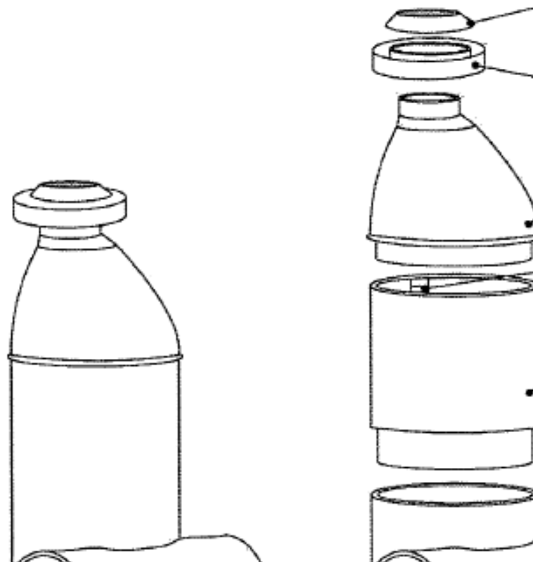
1 - база; 2 - шахта; 3 - лестница; 4 - конус-переход (горловина); 5 - форма для железобетонной плиты под люк; 6 - люк
