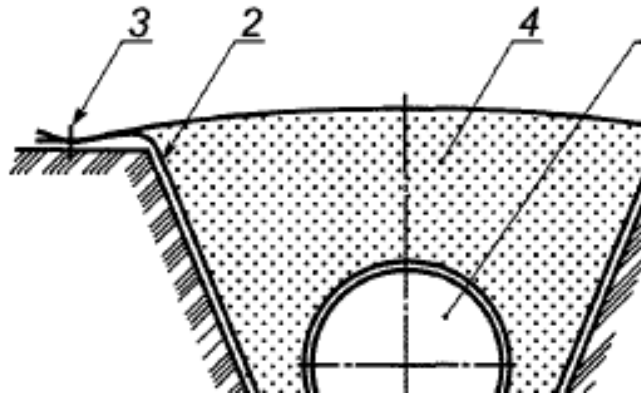
1 - трубопровод; 2 - полотнище из НСМ; 3 - металлический штырь; 4 - грунт засыпки Рисунок 6.10 - Способ балластировки трубопроводов грунтом засыпки с использованием НСМ при прокладке в песчаных грунтах
