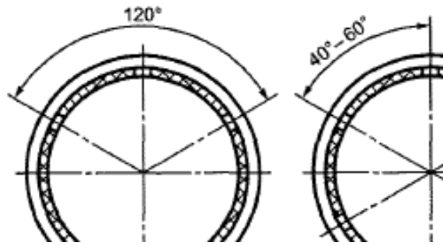
а - для труб DN/OD 110-160 мм; б - для труб DN/OD 200-630 мм и DN/ID 200-600 мм
