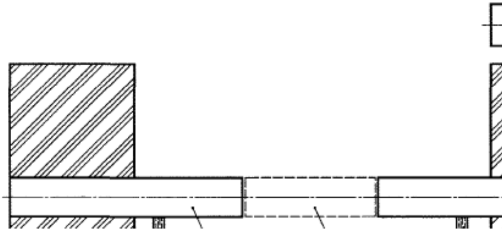
Рисунок 6.15 - Схема расположения трубной вставки между концами трубопровода
