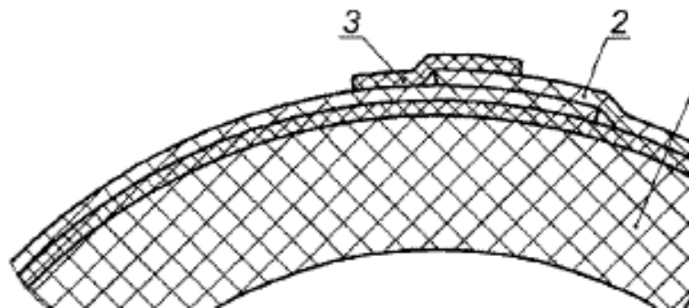
1 - труба; 2 - ТУЛ; 3 - замковая пластина
