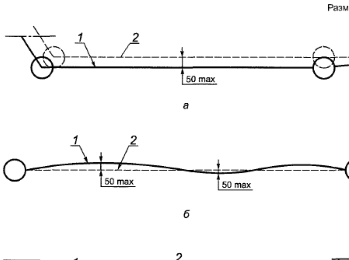
а - отклонение проектной трассы от фактической при изменении проектного положения колодцев; б - боковое отклонение трассы при сохранении проектного положения колодцев; в - отклонение трассы в вертикальном положении; 1 - фактическая трасса; 2 - проектная трасса
