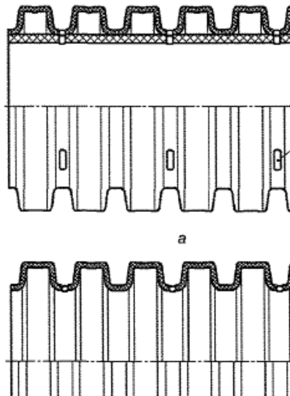
Рисунок 5.1 - Расположение водоприемных отверстий труб с двухслойной (а) и однослойной стенкой (б)
