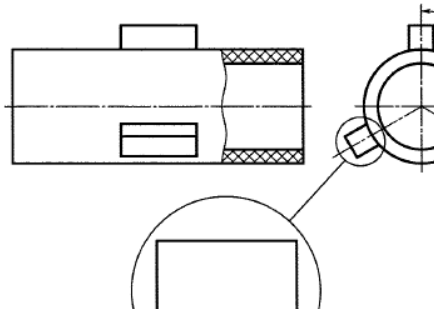
Рисунок 5.24 - Общий вид установки наварных элементов
