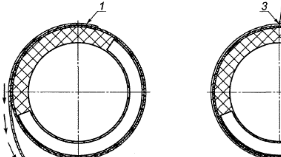
1 - место первоначальной фиксации ТУЛ; 2 - ТУЛ; 3 - место стыковки ТУЛ
