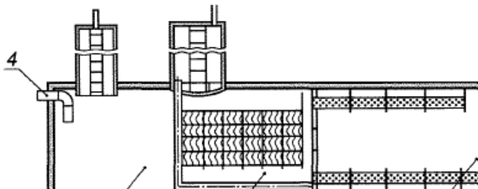
1 - пескоотделитель; 2 - маслобензоотделитель; 3 - сорбционный фильтр; 4 - подводящий патрубков; 5 - отводящий патрубков
