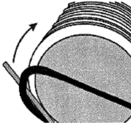
Рисунок 10.8 - Установка уплотнительного кольца при помощи двух монтировок
