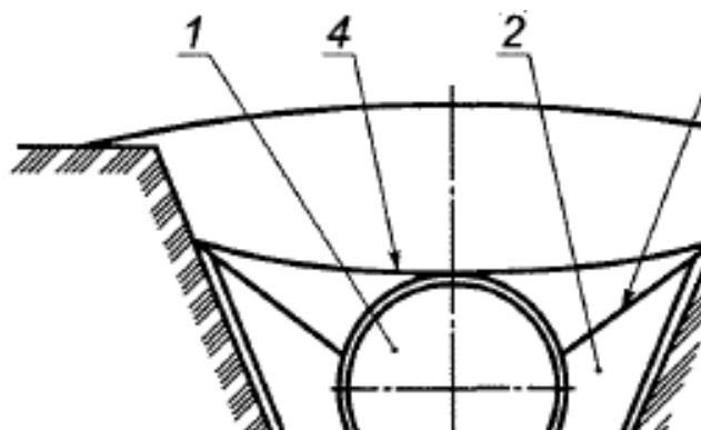
1 - трубопровод; 2 - контейнер из технической ткани; 3 - распорная рамка; 4 - грузовая лента Рисунок 6.12 - Балластировка трубопровода с помощью двух полимерных контейнеров
