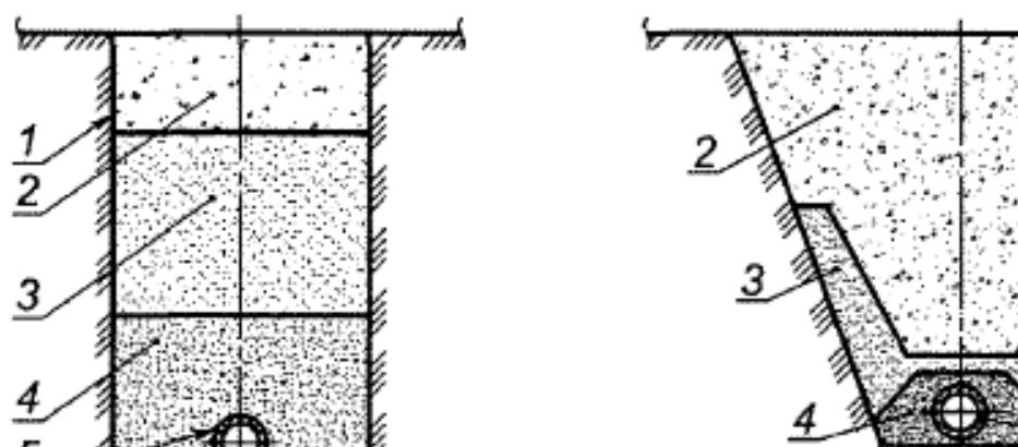
а - в траншее с вертикальными стенками; б - в траншее с откосами; 1 - контур траншеи; 2 - местный грунт; 3 - обратная засыпка траншеи разнозернистым песком; 4 - однослойная засыпка мелким щебнем; 5 - трубопровод
