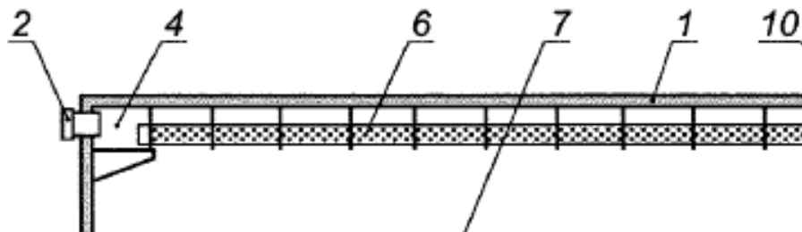
1 - корпус; 2 - подводящий патрубков; 3 - отводящий патрубков; 4 - приемная камера неочищенных стоков; 5 - приемная камера очищенных стоков; 6 - труба распределения потока; 7 - приемные трубы очищенных стоков; 8 - вентиляционная труба; 9 - лестница; 10 - шахта обслуживания
