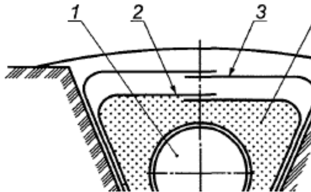
1 - трубопровод; 2 - полотнище из НСМ; 3 - бандаж; 4 - грунт засыпки Рисунок 6.11 - Способ балластировки трубопроводов грунтом засыпки с использованием НСМ при прокладке в глинистых и суглинистых грунтах
